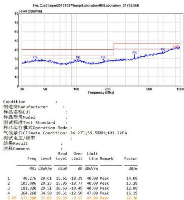
图 5-5 RE 测试水平方向
