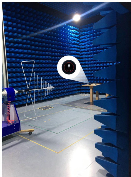
图 5-4 RE 测试图
