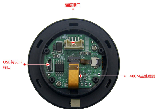
图 1-2 硬件配置图
