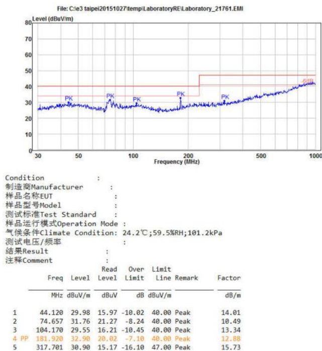
图 5-6 RE 测试垂直方向
