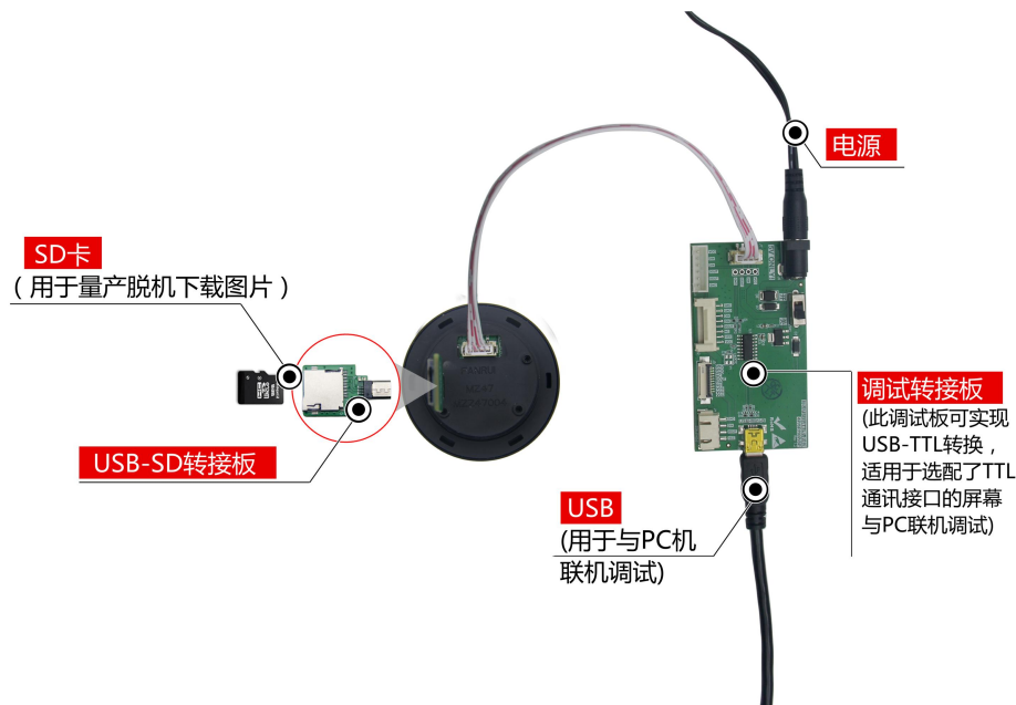
图 1-3 TTL 调试工具图
